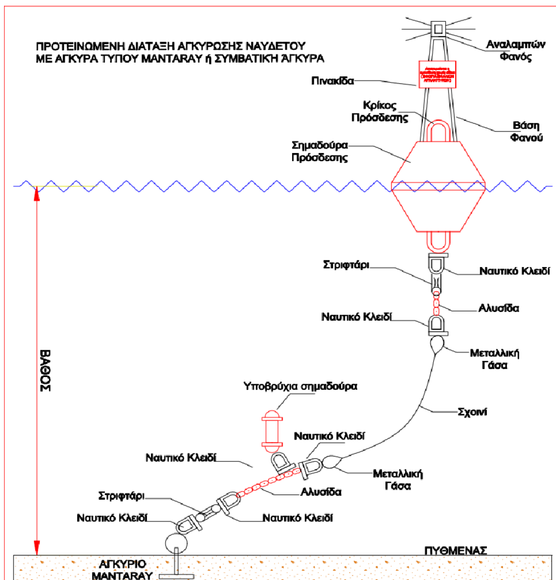
ΣΧΗΜΑ 1 (ΔΙΑΤΑΞΗ ΑΓΚΥΡΩΣΗΣ ΝΑΥΔΕΤΟΥ)
