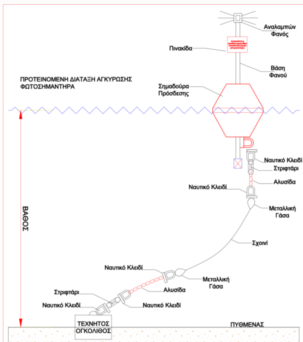
ΣΧΗΜΑ 2 (ΣΧΗΜΑΤΙΚΗ ΔΙΑΤΑΞΗ ΑΓΚΥΡΩΣΗΣ ΦΩΤΟΣΗΜΑΝΤΗΡΑ)
